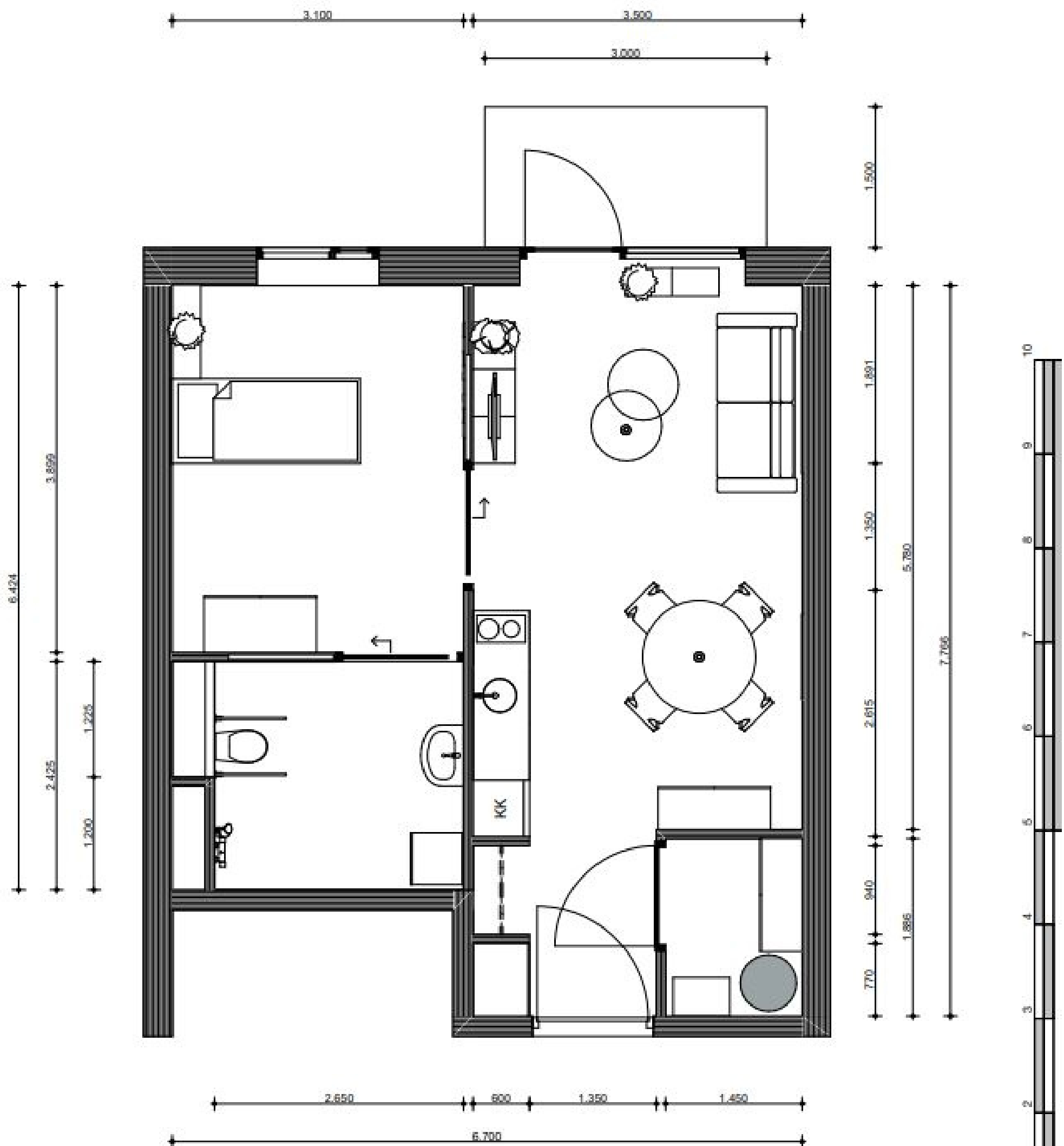
Het Laar | Laarstede 2KA Appartement type A, 6.70 x 7.77 m De materialen en de maatvoering op deze tekening zijn indicatief. Er kunnen geen rechten aan worden ontleend.
